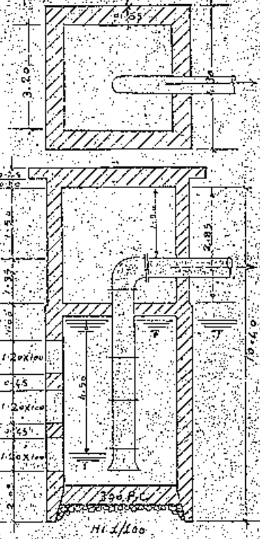
Gölcük keson dairesinin Planı ve mekeli
